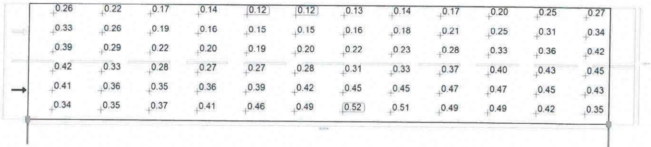
Observator 1: Valoarea de întreținere, densitatea luminii cu carosabil uscat [ \text{cd}/\text{m}^2 ] (Raster valoric)
