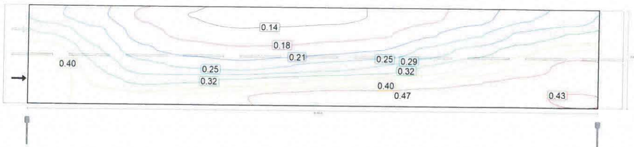
Observator 1: Valoarea de întreținere, densitatea luminii cu carosabil uscat [ \text{cd/m}^2 ] (Linii Isolux)
