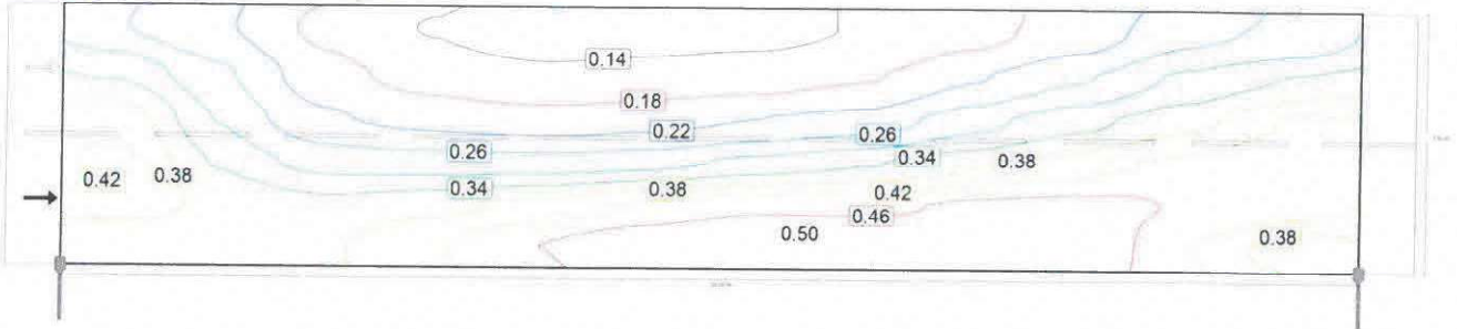
Observator 1: Valoarea de întreținere, densitatea luminii cu carosabil uscat [ \text{cd}/\text{m}^2 ] (Linii Isolux)
